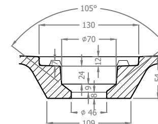
DETAGLIO SCARICO 1:5
