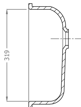
B-B
