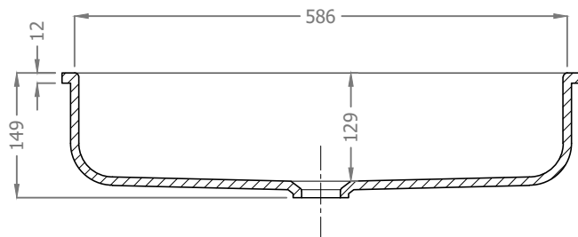
A-A
