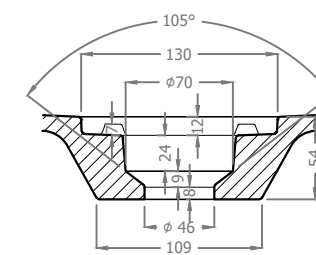
DETTAGLIO SCARICO 1:5
