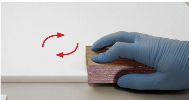
3. Carteggiare la zona interessata al graffio il tampone in legno (C) e la carta Grana 800 (A), poi con la carta Grana 1200 (B) seguendo il senso indicato.
